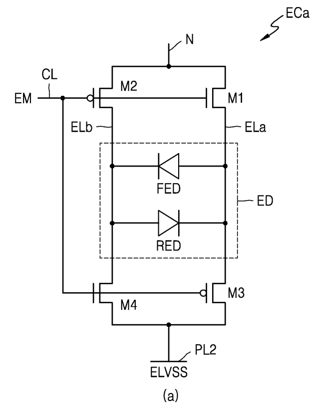
도면5
